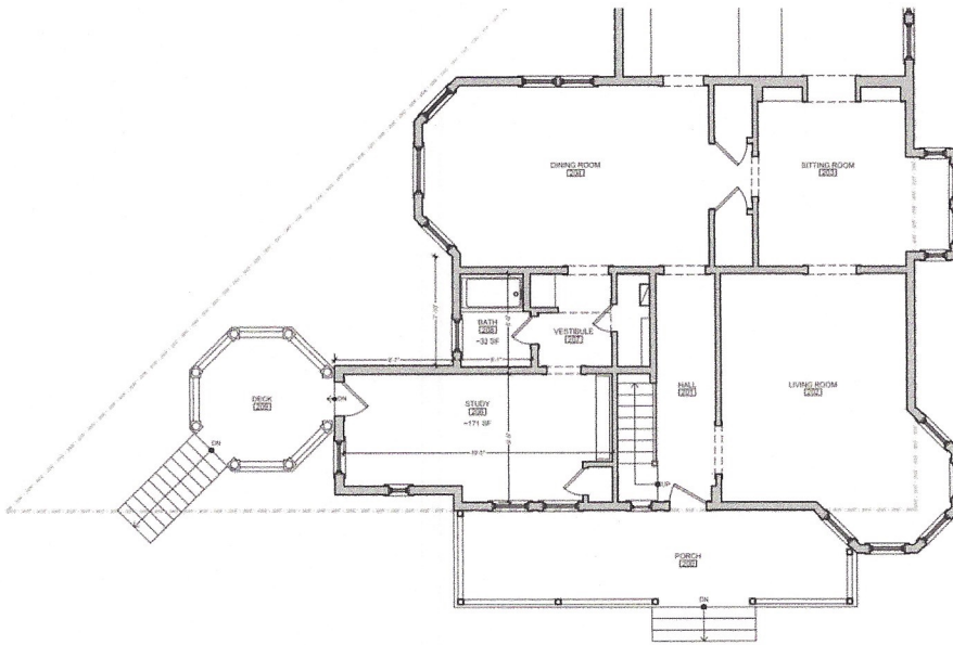
EXISTING PLAN SCALE: 1/8" = 1'-0"
