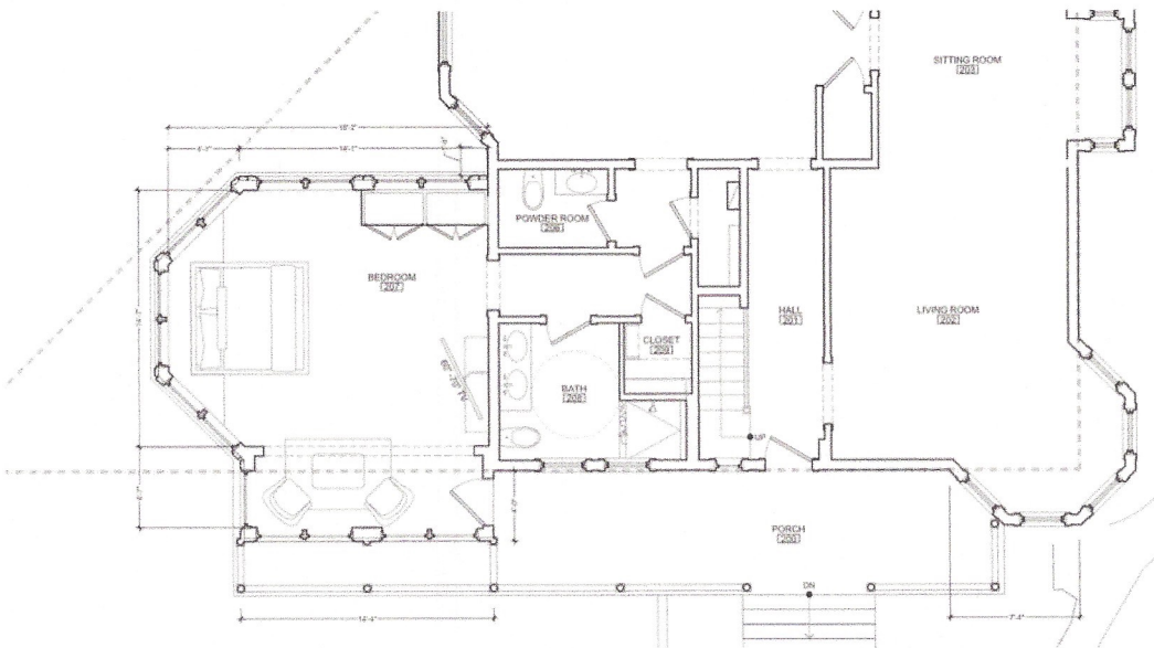
01 OPTION 2 SCALE: 1/8" = 1'-0"
